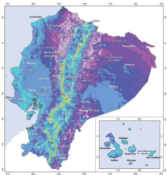
ATLAS EOLICO DEL ECUADOR Velocidad Media Anual del Viento a 80 m de Altura sobre el Suelo
