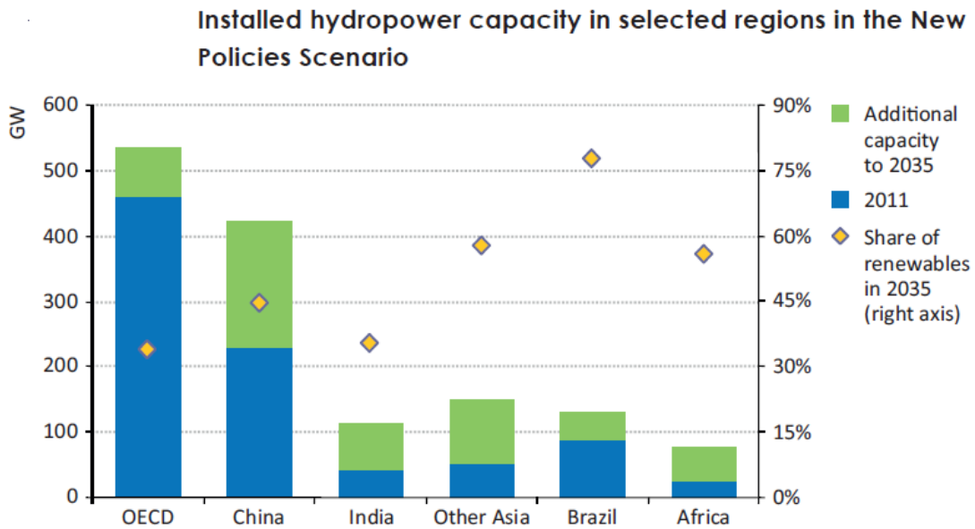
Fig.1. Proyección de la Capacidad instalada Hidroeléctrica en el Mundo
